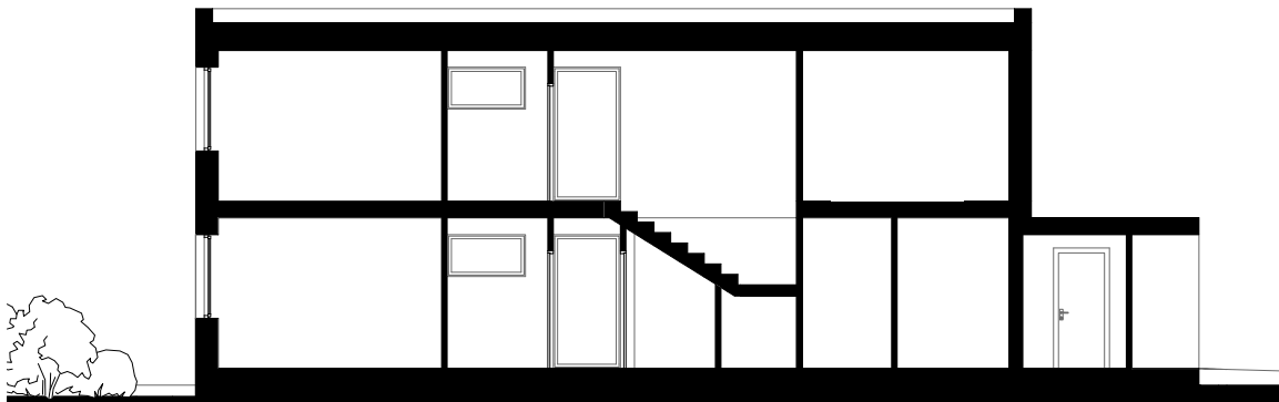
■ ■ ŘEZ_1:150
